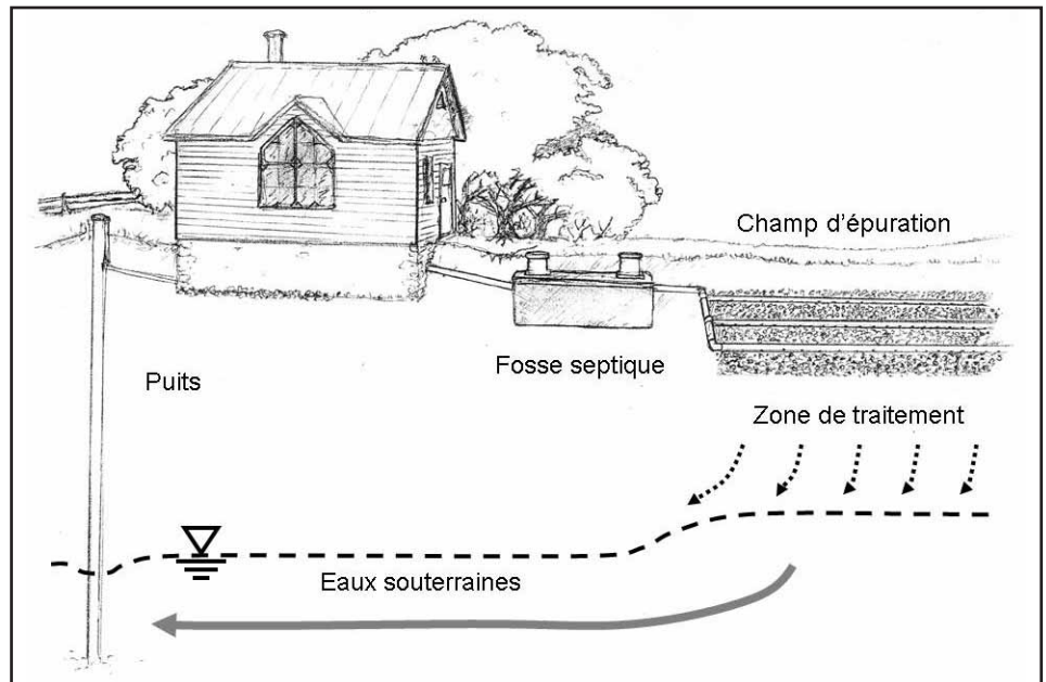
Figure 1 Recyclage des eaux usées par une installation autonome
